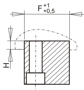
SECCION B-B SECTION B-B
