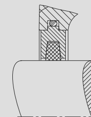
Obturación de fieltro
