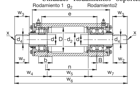
VRE3...C
