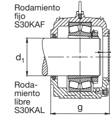
Ejecución A desde S3044K
