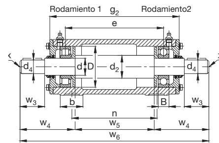
VRE3...B
