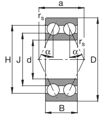
32B, 33B Angulo de contacto \alpha = 25^\circ
