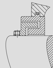
Obturación de laberinto axial
