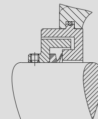
Obturación de laberinto + Taconite axial
