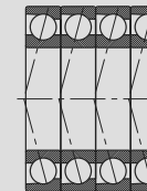
QTT Disposición en Tándem
