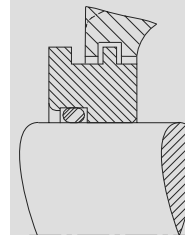
Obturación de laberinto radial
