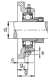
F162
