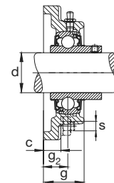
F562
