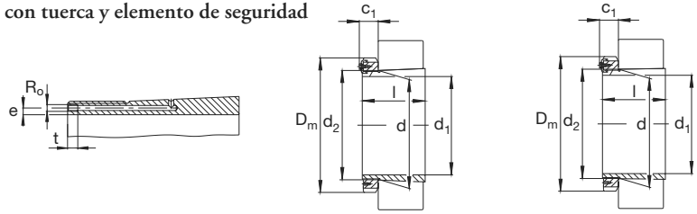
Manguito de montaje hidráulico (sufijo HG)
