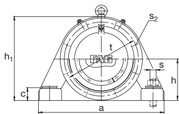
Ver páginas 663 y 664 para la sección de los soportes BND con rodamientos con agujero cilíndrico.
