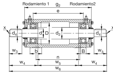
VRE3...A
